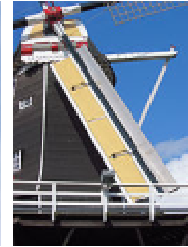
Aile mixte avec bord d'attaque Van Bussel (à droite) et système Ter Have (à gauche), Winterswijk, Pays-Bas.
