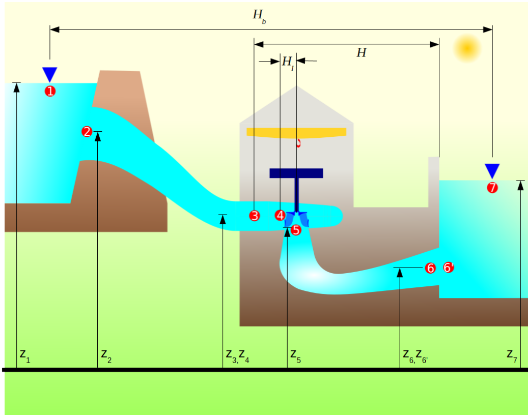
Coupe d'une installation hydroélectrique
