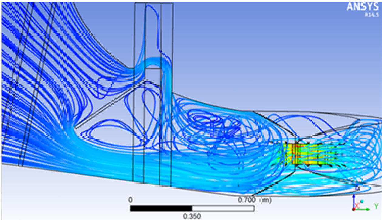
La grille à poisson perturbe de façon considérable les écoulements, réduit les performances et crée de la nuisance additionnelle pour les poissons qui ne sont pas capturés
