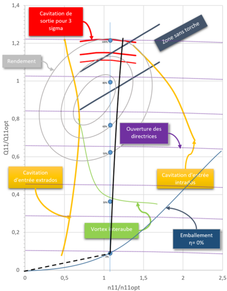
Colline de rendement typique
