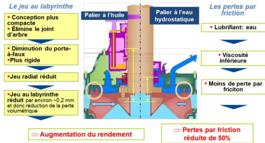
Avantages du palier hydrostatique à l'eau
