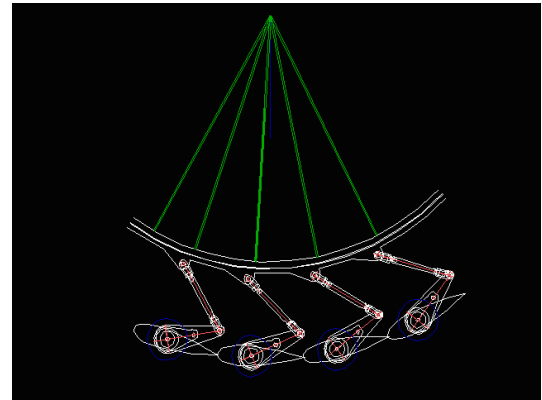
Synchronisation de l'ouverture des directrices
