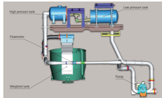
Schéma d'une plate-forme d'essai de modèle réduit
