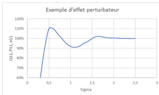
L'effet perturbateur de la cavitation peut affecter : le rendement, le débit, la puissance et la vitesse d'emballement
