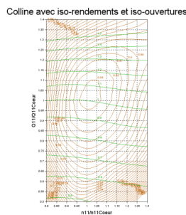
Colline classique avec iso-rendements et iso-ouvertures
