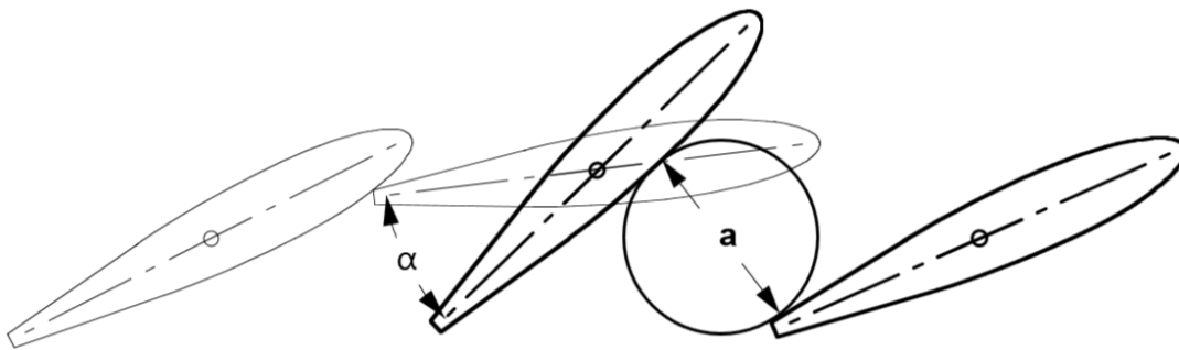
Position fermée: \alpha = 0^\circ ou a = 0 mm
