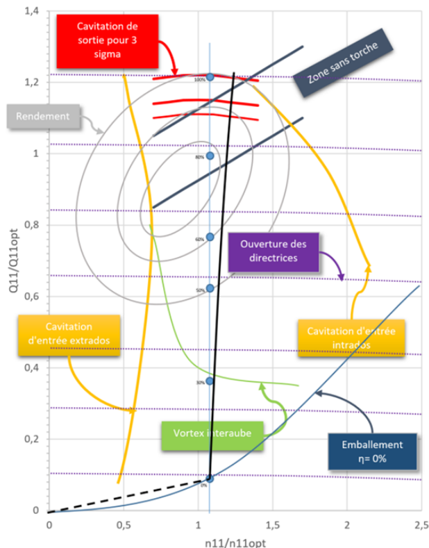
Une prise de charge en turbine
