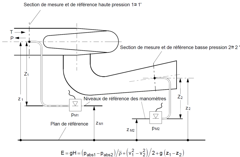
Sections de mesure haute et basse pression pour l'énergie nette selon CEI60193
