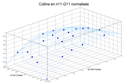
Colline en n11-Q11 normalisée
