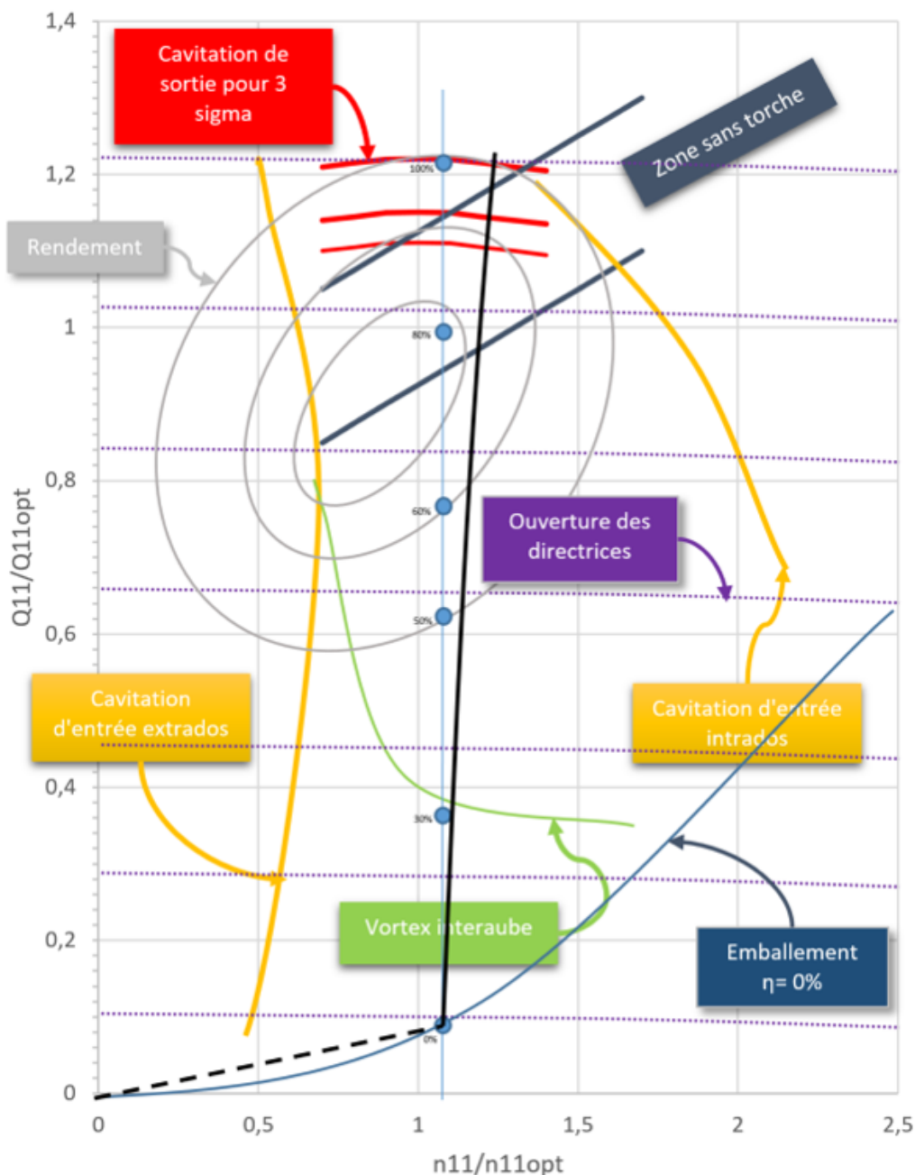
Colline de rendement typique
