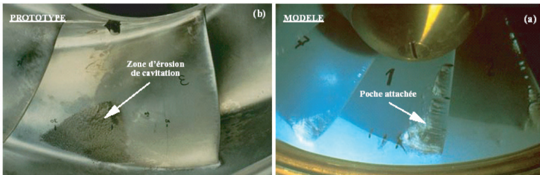
Figure 1.5 – (a) : Développement de la cavitation d'entrée dans un modèle de pompe d'accumulation. (b) : dégâts d'érosion sur le prototype après 400 h de fonctionnement Farhat [1994]
