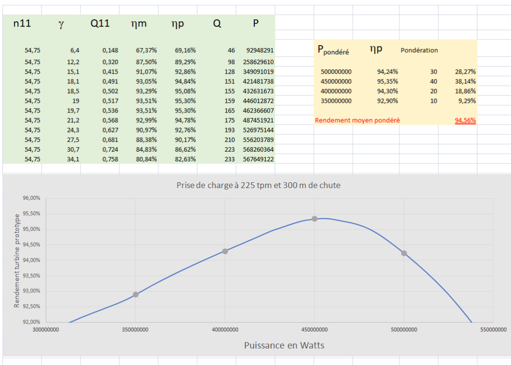
Prise de charge
