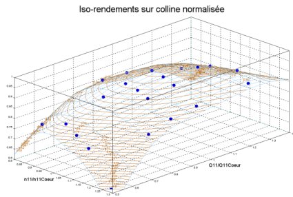
Colline avec iso-rendements - Vue isométrique
