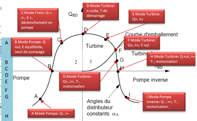
Figure 114 – Diagramme des différents modes de fonctionnement Pour une ouverture de directrice donnée.
