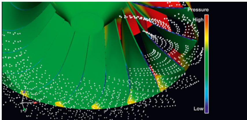
Aération par le bord de fuite des aubes
