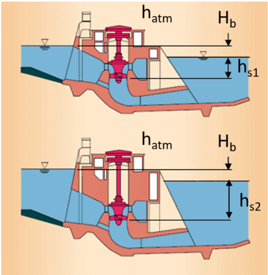
Une diminution de h_s (ou augmentation de l'enfoncement) réduit la cavitation mais augmente les coûts du civil.
