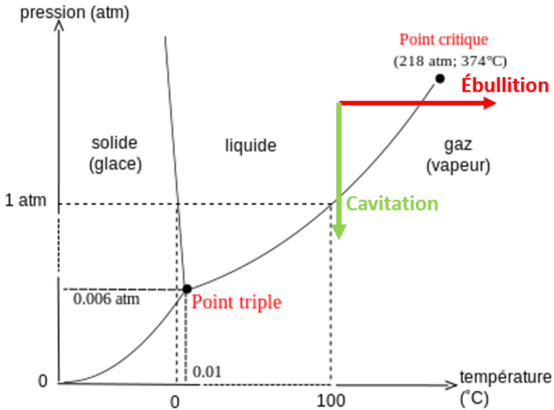
Diagramme Pression-Température
