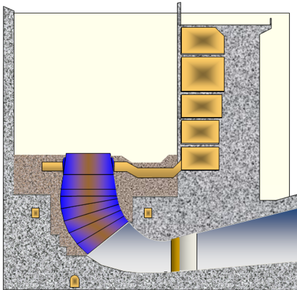
Montage des pièces encastrées
