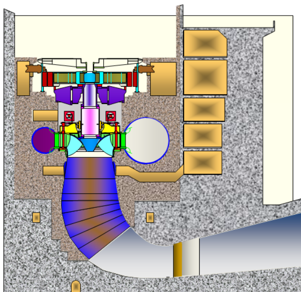
Montage de l'alterneur
