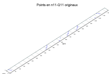
Points originaux distribués dans le domaine d'interpolation
