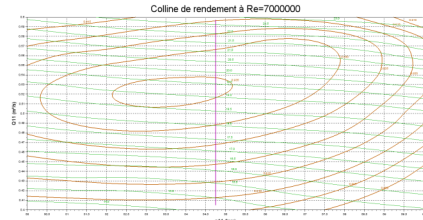
Colline de rendement
