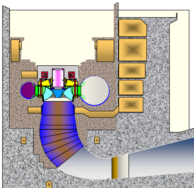
Les directrices puis le flasque supérieur sont montés, suivis du mécanisme de vannage
