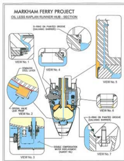
Moyeu de Kaplan sans huile
