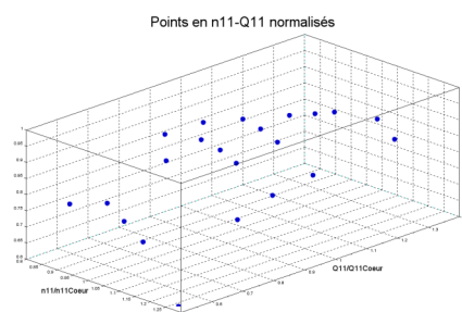
Points normalisés distribués dans le domaine d'interpolation
