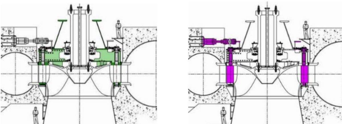
À gauche : parties fixes du distributeur À droite : parties mobiles du distributeur
