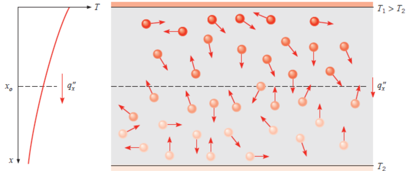
Schématisation de la conduction dans un fluide au repos
