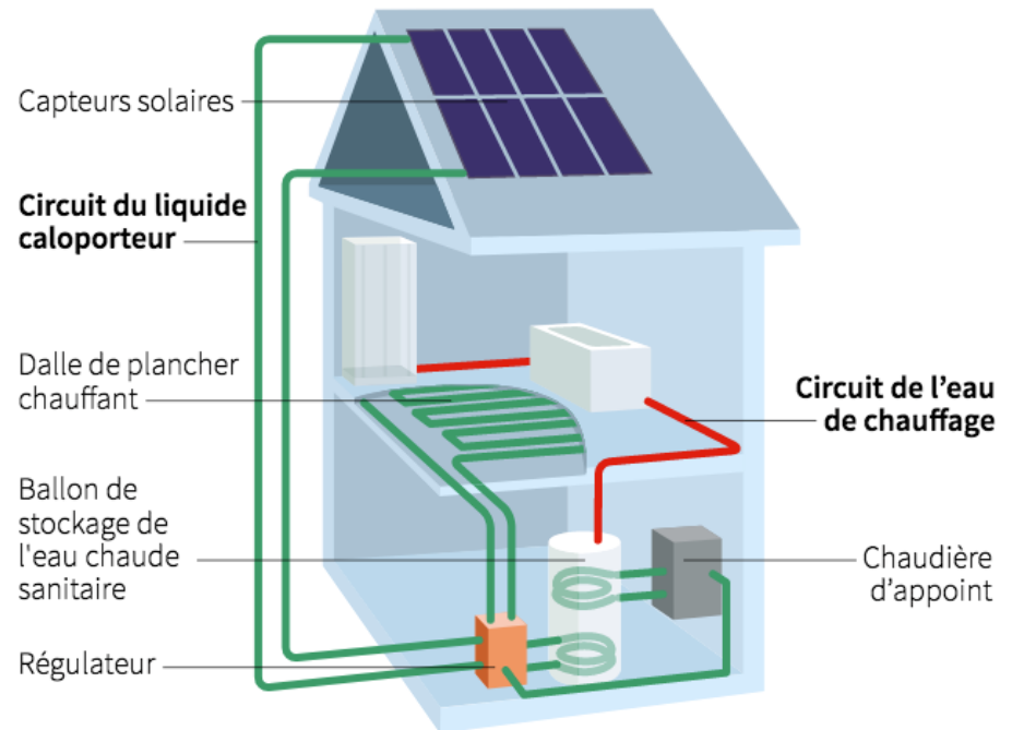
PRINCIPE DU SSC SOLAIRE DIRECT
